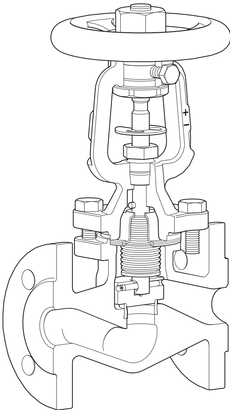
图1 BSAT图示
